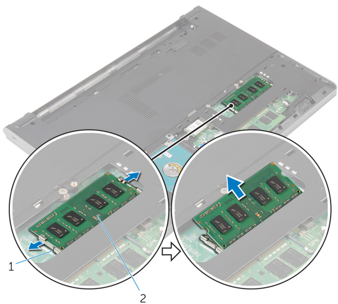
1 固定クリップ (2)
